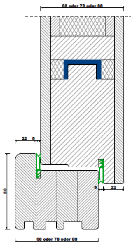
waagerechter Schnitt glattes Türblatt
