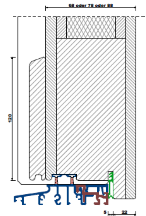
senkrechter Schnitt glattes Türblatt
