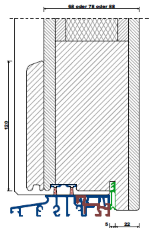
senkrechter Schnitt glattes Türblatt
