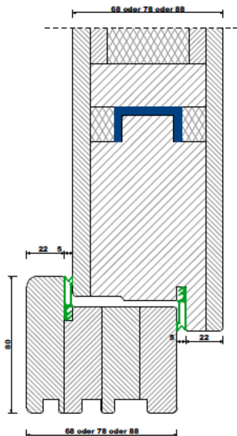
waagerechter Schnitt glattes Türblatt
